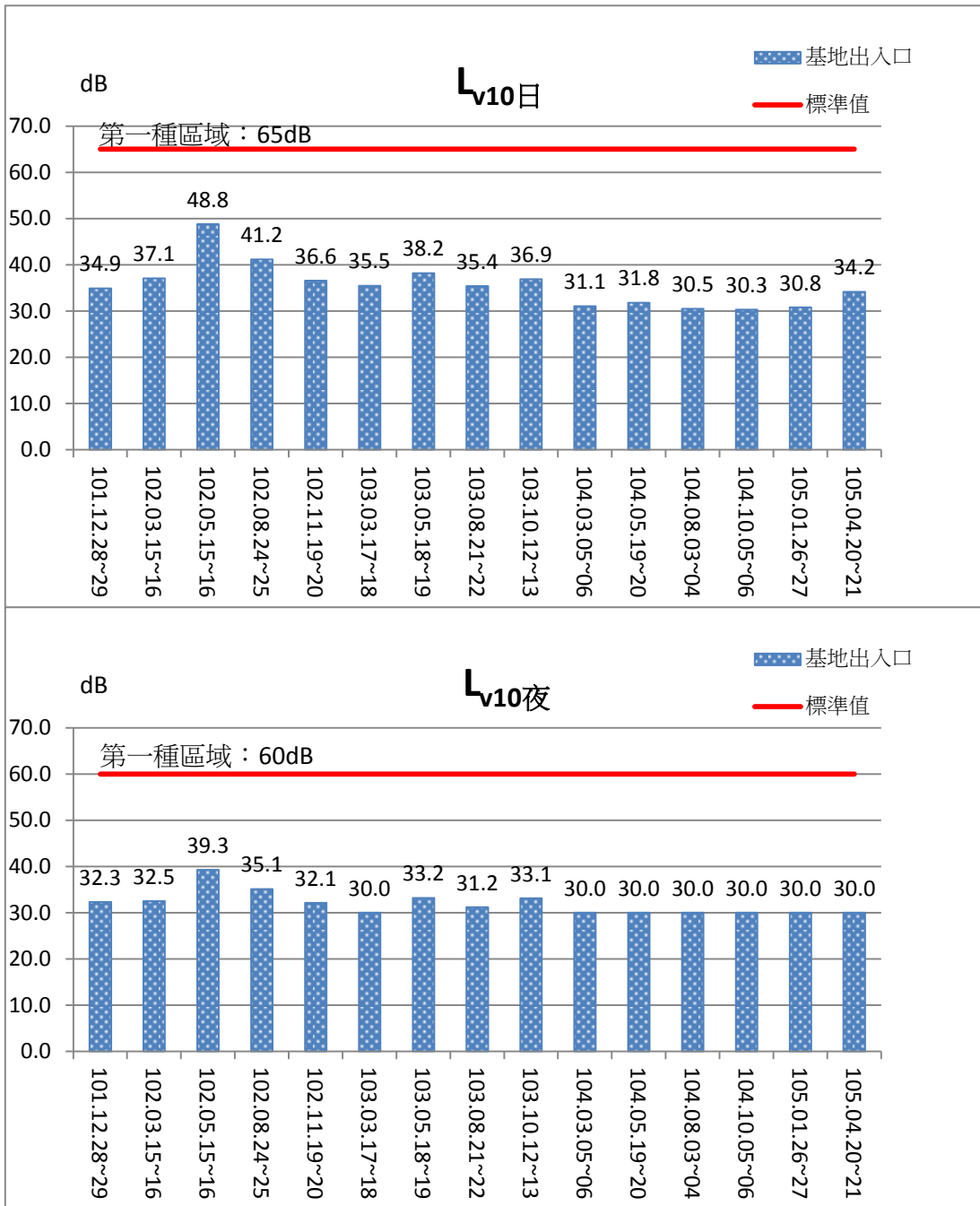
圖 2.2-3 基地出入口振動監測結果比較圖
