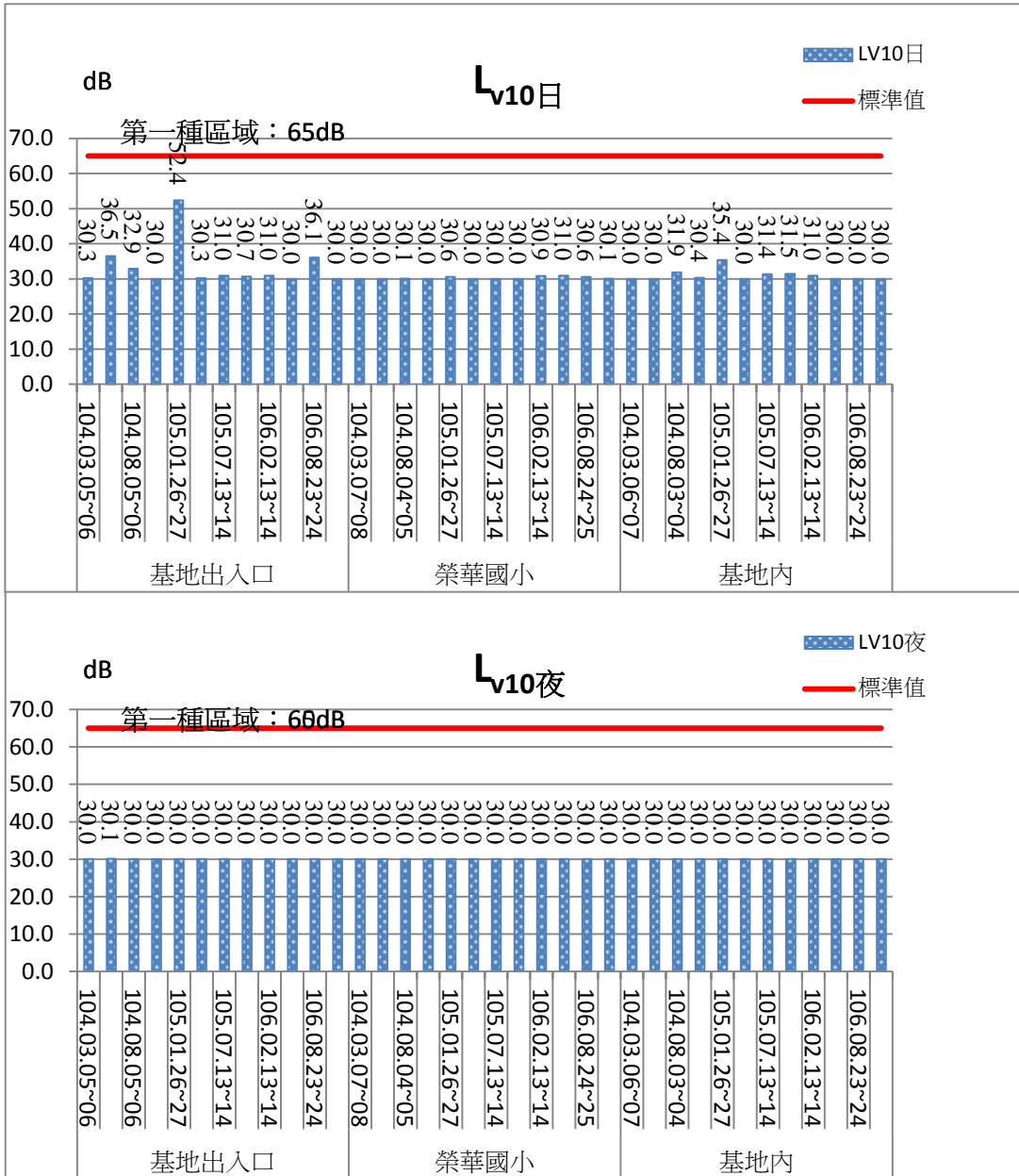
圖 2.2-3 基地出入口、榮華國小及基地內振動監測結果比較圖
