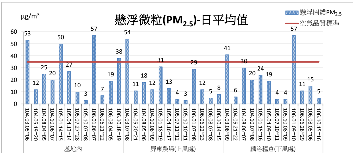
圖 2.1-15 PM 2.5 各測點日平均監測結果比較圖
