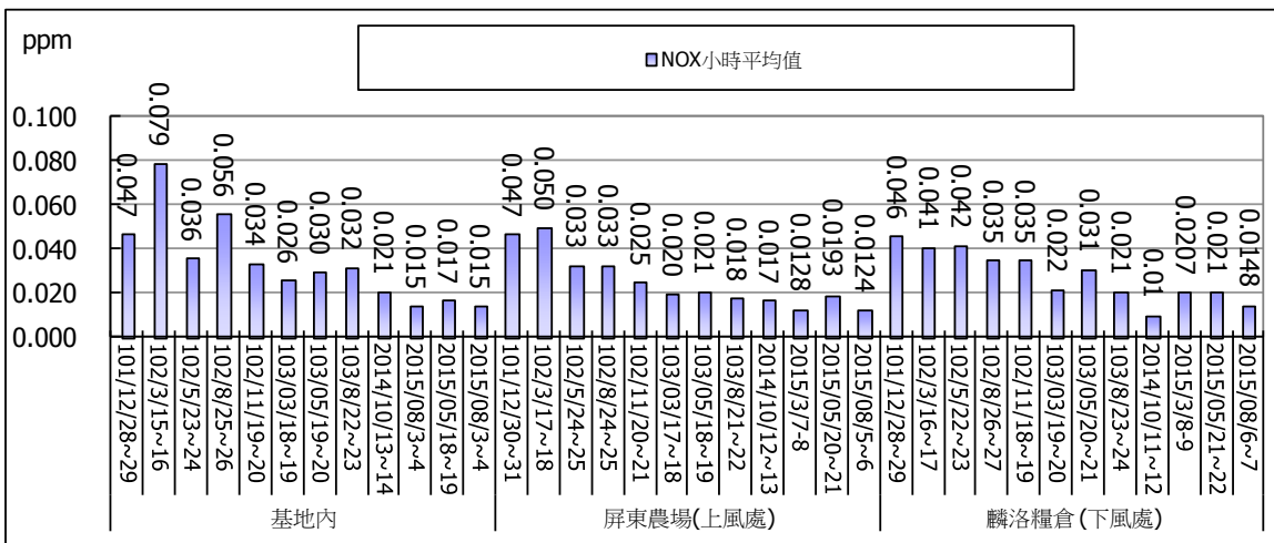
圖 2.1-8 二氧化氮各測點最高小時平均值監測結果比較圖
