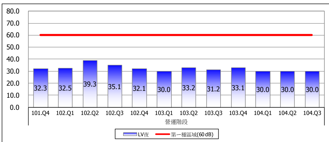
圖 2.2-3 基地出入口振動監測結果比較圖
