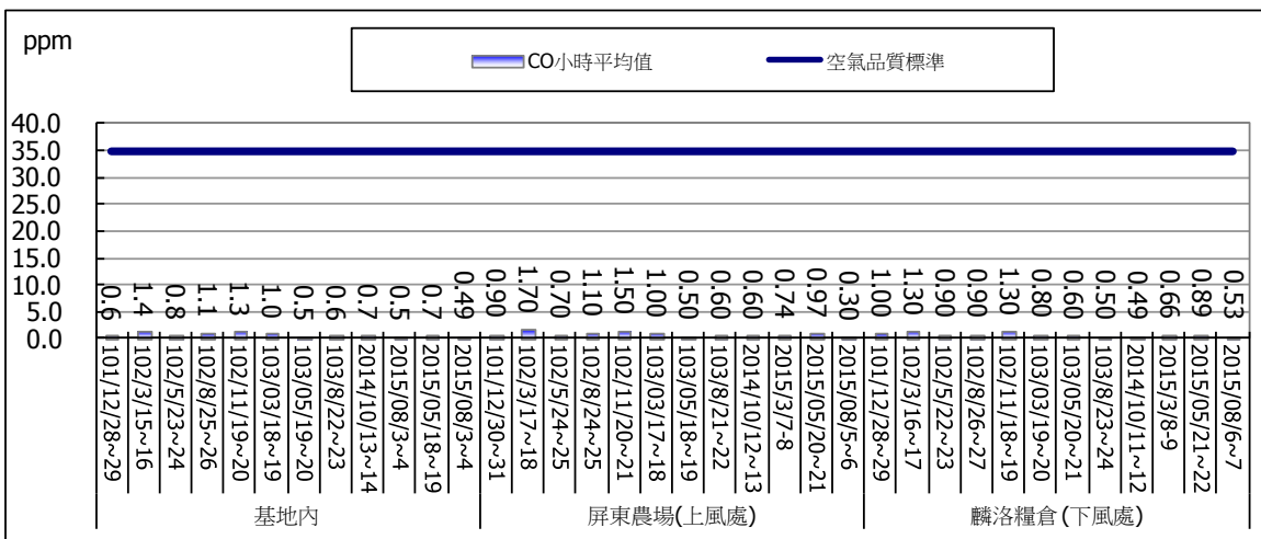
圖 2.1-11 一氧化碳各測點最高八小時平均值監測結果比較圖
