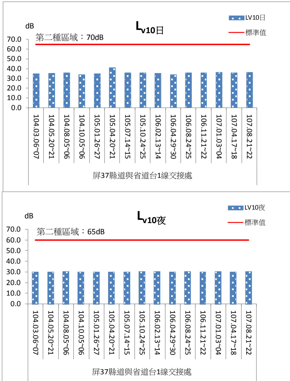
圖 2.2-4 屏 37 縣道與省道台 1 線交接處振動監測結果比較圖
