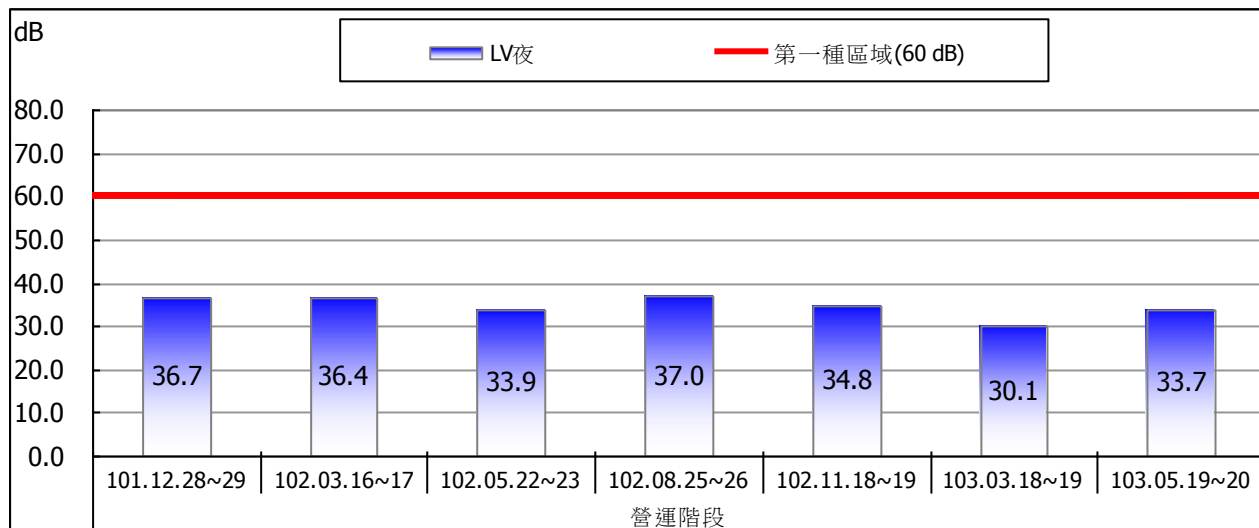
圖 2.2-4 屏 37 鄉道與台 1 省道交接處振動監測結果比較圖
