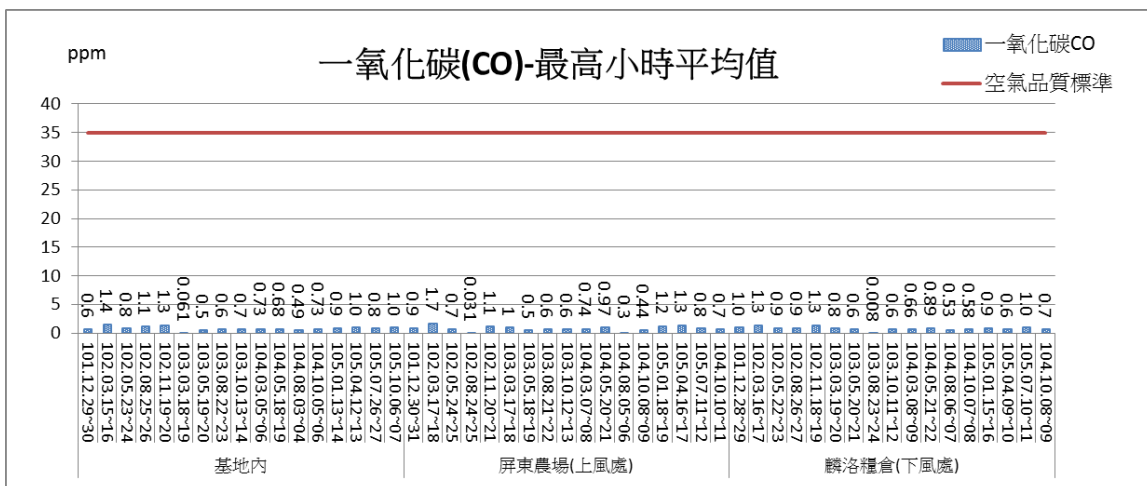
圖 2.1-12 一氧化碳各測點最高小時平均值監測結果比較圖
